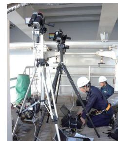
神戸大学との共同研究（鋼床版の疲労点検）
