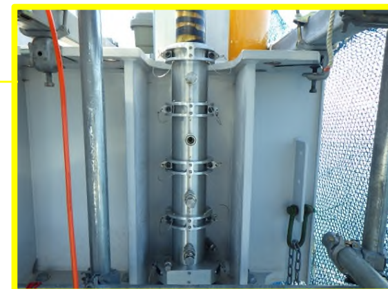
ハンガーロープ防食内部充填工法
