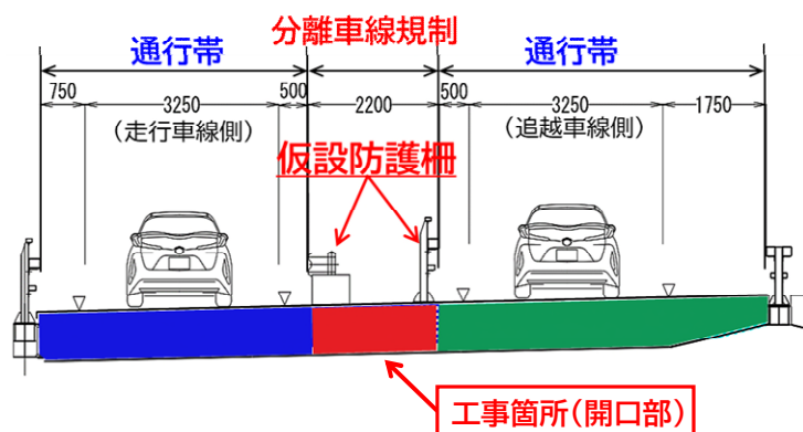
規制概略断面図
