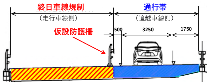
①④⑦走行車線規制概略断面図
