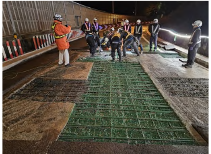
床版断面修復
