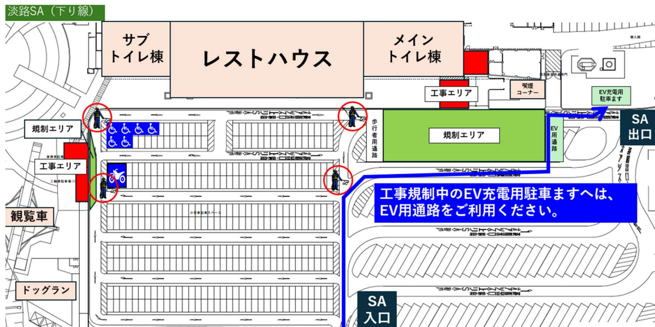
(平日日中の作業時) 淡路サービスエリア(下り線) 規制図
