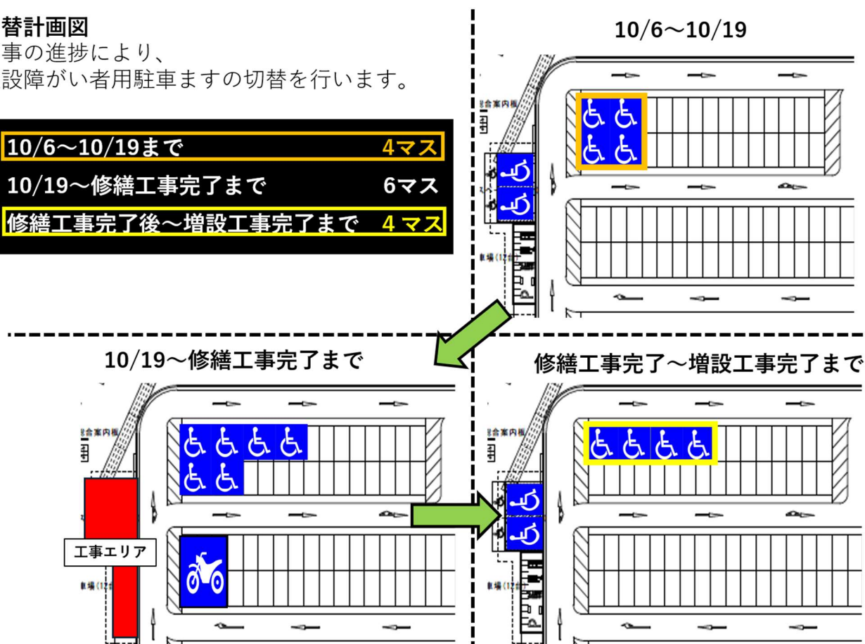
仮設障がい者用駐車スペース等の切替計画図
