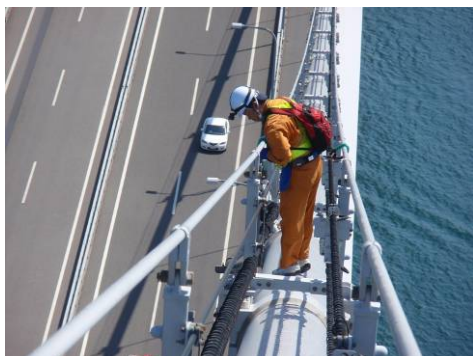
長大橋(吊橋ケーブル)点検状況 (一般国道 317 号 来島海峡大橋)
