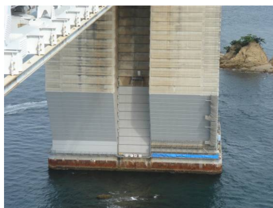
吊橋アンカレイジの防食塗装の状況 (一般国道 30 号 南北備讃瀬戸大橋)
