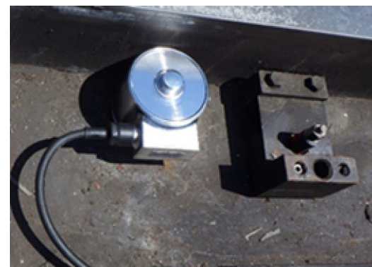
軸重計ロードセル (補修前)
