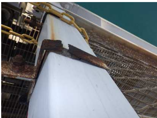
管理用通路支柱側面パネル (補修前)
