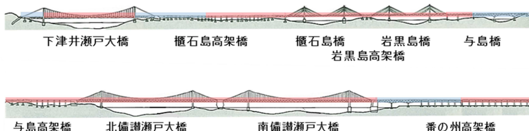
平成 29 年度末における瀬戸大橋耐震補強工事進捗状況
