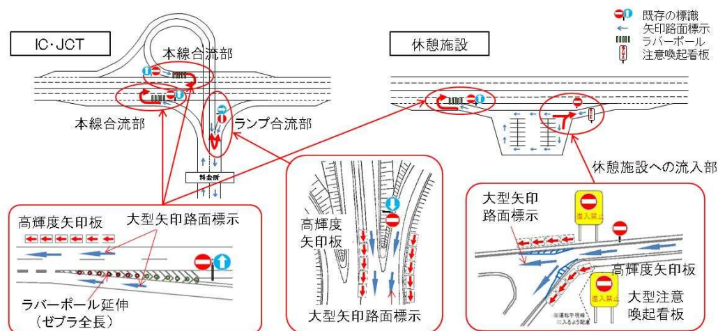
《平成27年4月に公表した対策の基本パターン(イメージ)》
