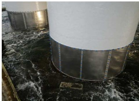
2P 飛沫部塗装、干満部チタンカバー設置状況 (一般国道 28 号 大鳴門橋)
