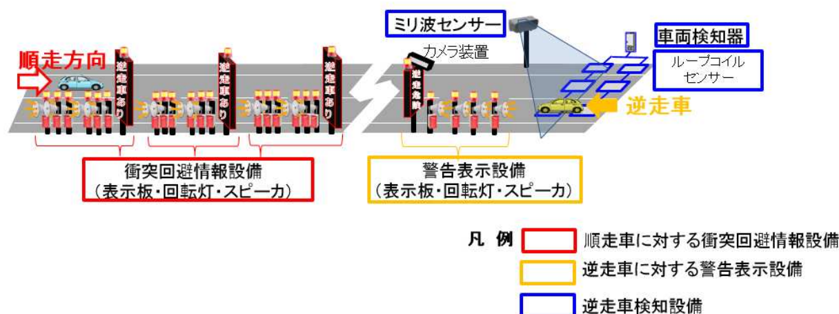
逆走対策システム(イメージ)
