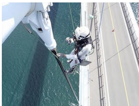
長大橋技術支援 (広島県道路公社/豊島大橋)
