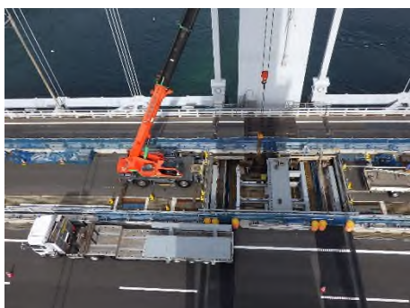
大鳴門橋 伸縮装置更新工事 (神戸淡路鳴門自動車道)
