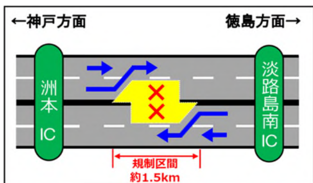
追越車線規制概要図
