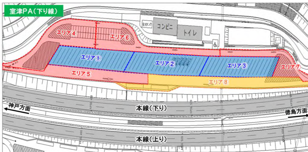
室津パーキングエリア PA(下り線) 工事エリア分割図
