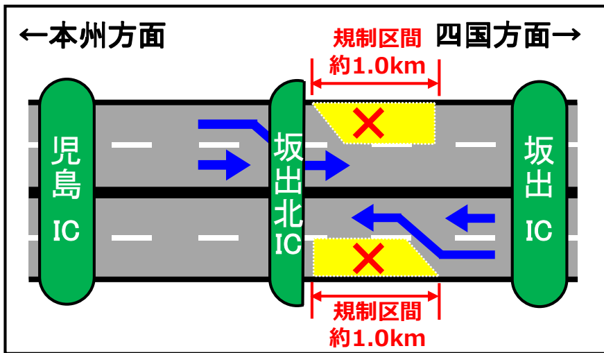
走行車線規制概要図
