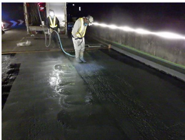
床版防水層の施工
