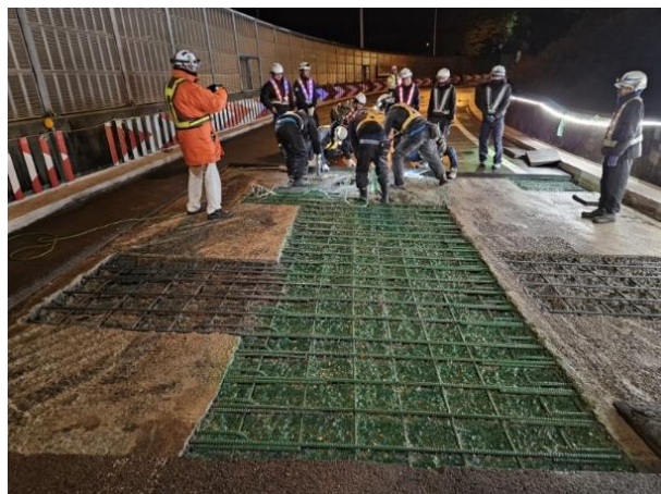
コンクリート床版の断面修復
