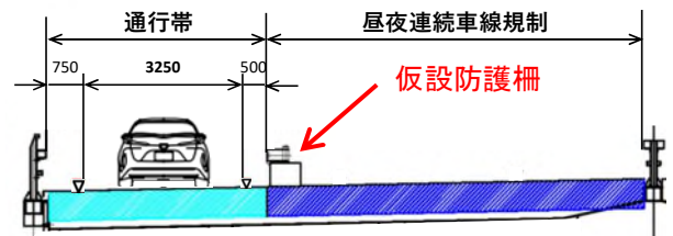
追越車線規制概略断面図
