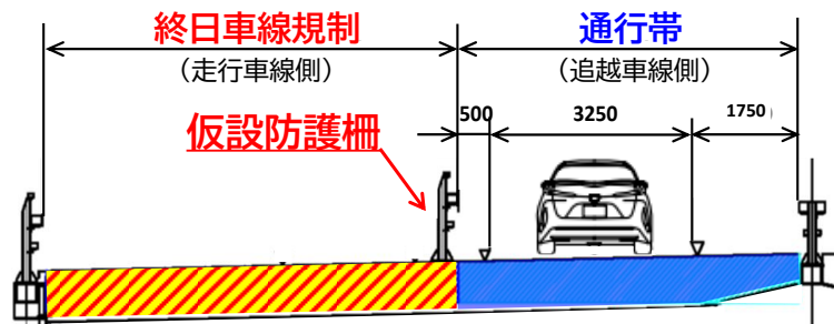
①④ 走行車線規制概略断面図
