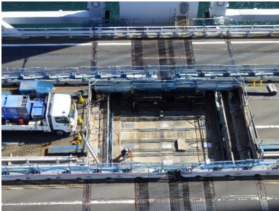
③(旧)大型伸縮装置撤去状況
