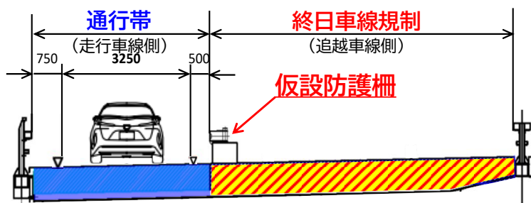
②⑥ 追越車線規制概略断面図
