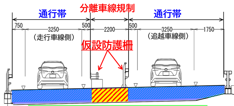
③⑤ 分離車線規制概略断面図
